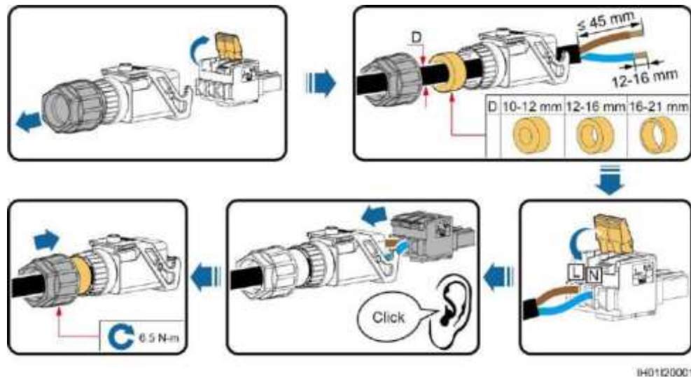
5-8. ábra AC csatlakozó összeszerelése (kéteres vezeték)
