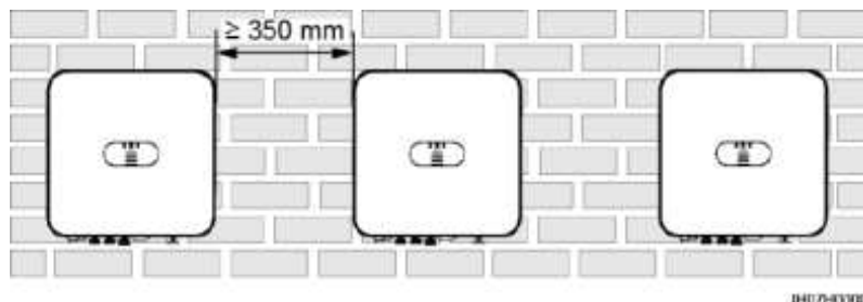
4-3. ábra Vízszintes szerelési mód (ajánlott)
