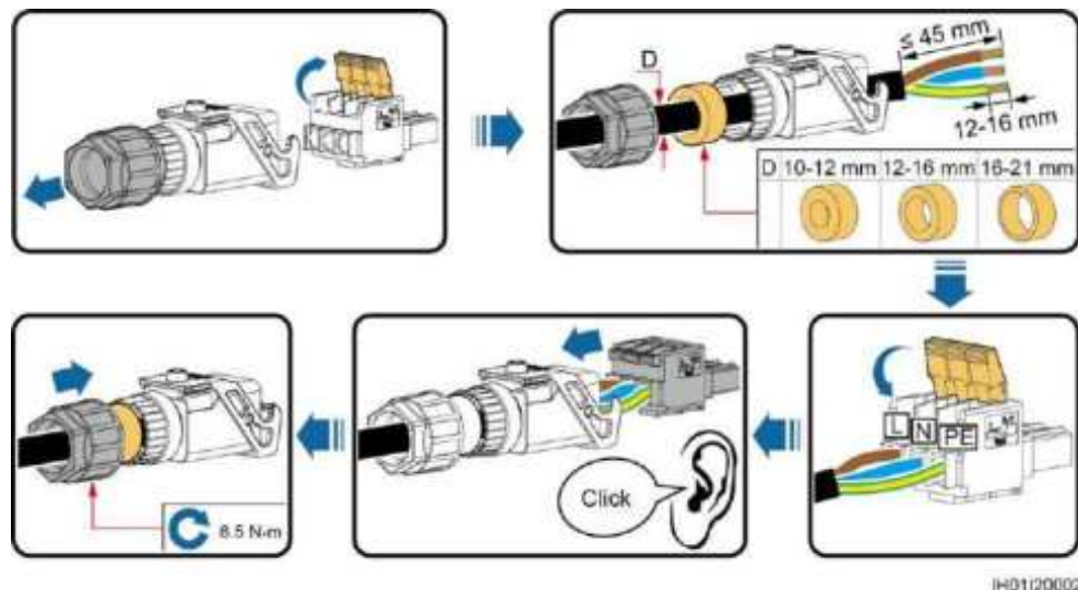
5-7. ábra AC csatlakozó összeszerelése (háromeres vezeték)
